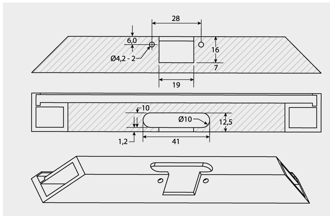
Разметка позиций крепления для чашки петли
