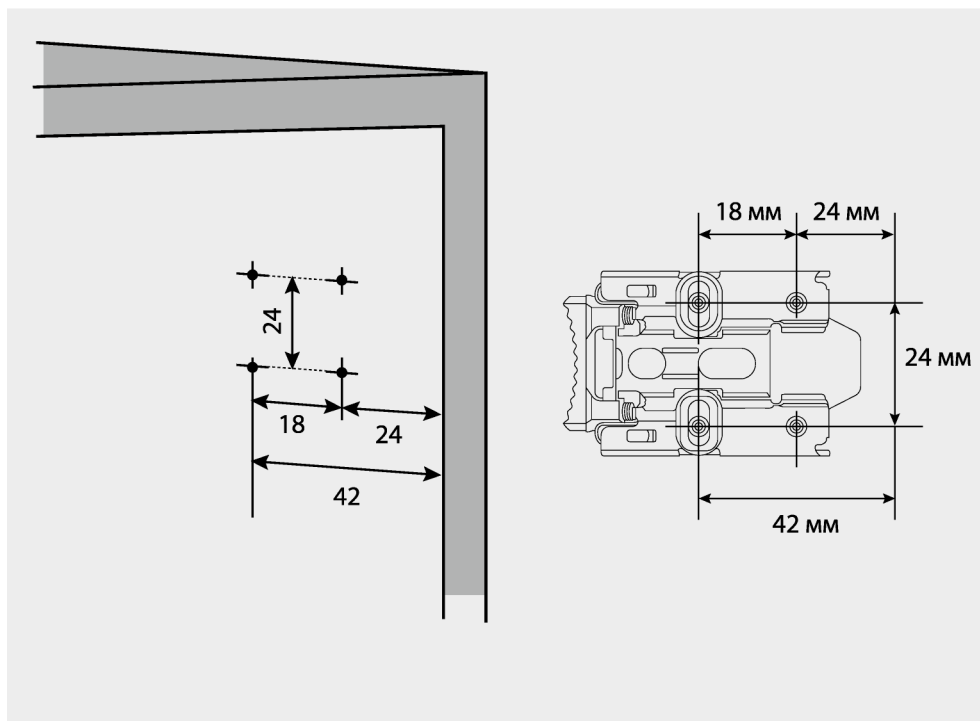
Разметка позиций крепления для монтажной планки
